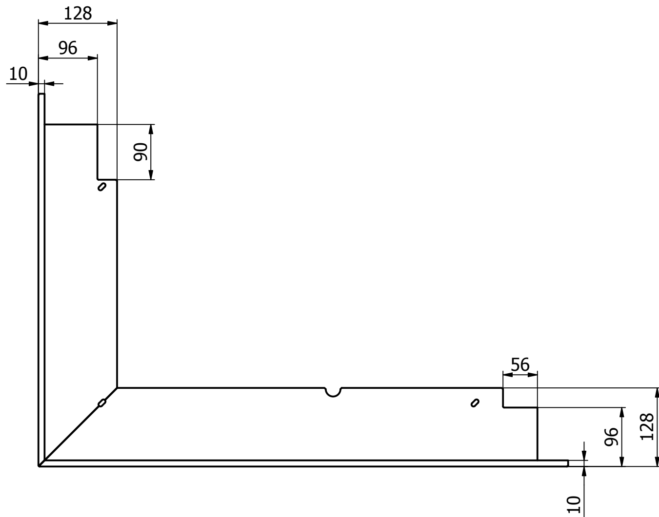
Maskownica 50 głęboka
